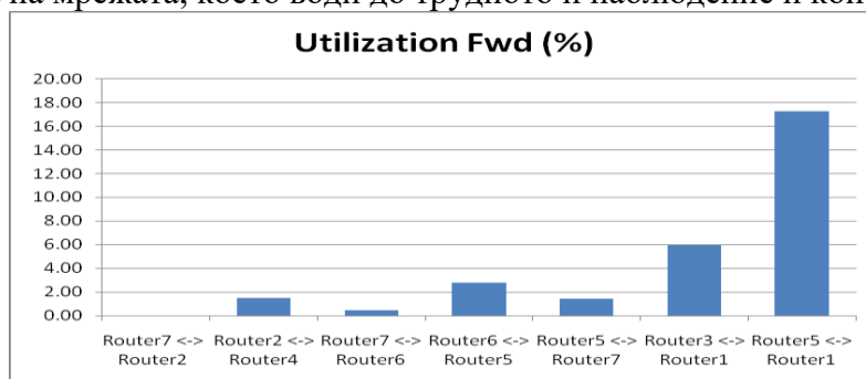
Фиг.11. Използването на 1Gbps връзки в права посока при 75% натоварване на връзката между R7 и R2 и 25% между R5 и R1.
