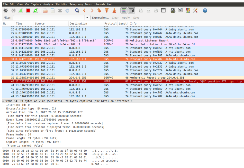
Фиг. 3 Общ екранен изглед на програмата Wireshark
