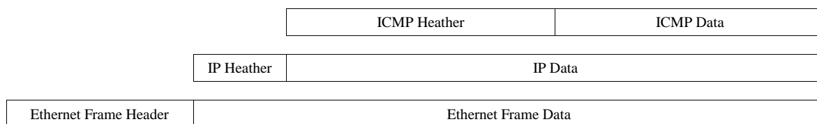
Фиг. 1.a. Енкапсулация на ICMP пакета в IP и Ethernet рамката.
